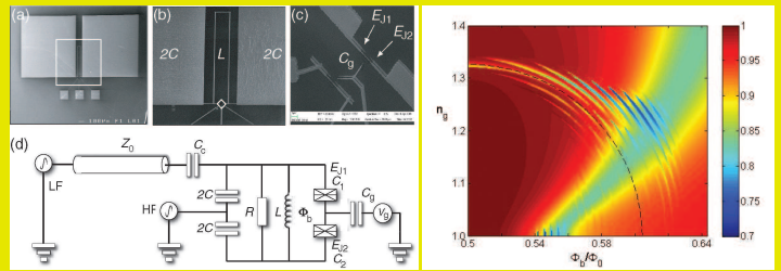
Sähköinen piiri, jossa suprajohtavia liittoksia ja sille laskettu heijastusspektri
