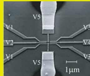
Kaksi rinnakkaista kvanttipistettä ja niitä säätelevät elektrodit
